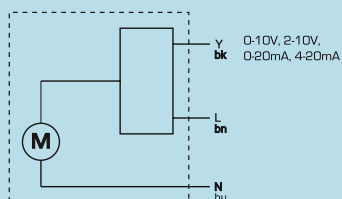
Servopohony řady ARA659
