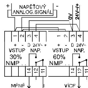
Zapojení dvou NMP .. na jeden analogový signál - ovládání pohonu.
