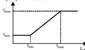
Obr. 1 Použití f_{min} a f_{max} pro omezení výstupního kmitočtu Výstupní kmitočet
