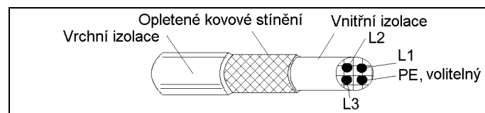
Obr. 8 Účinné stínění motorového kabelu (např. Ölflex-Servo-FD 780 CP, Lappkabel nebo MCMK, NK kabely)
