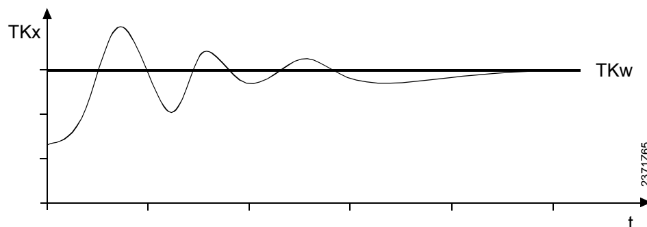
Rychlé vyregulování modulovaného hořáku
