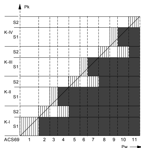
Pořadí spínání stupňů – sériově 2k
