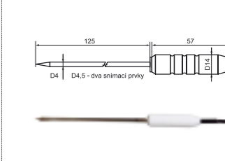
2061-200/E (-30 až +200 °C)
