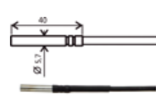
Pt100TG8/E (-80 až +200°C)
